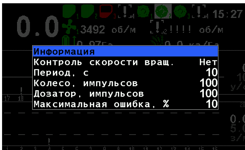
РИСУНОК 20 ПАРАМЕТРЫ ДОЗАТОРА
