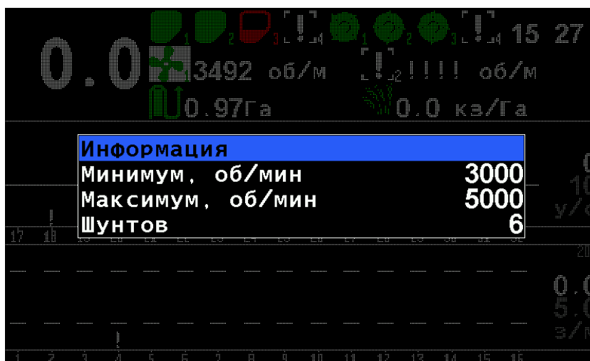
РИСУНОК 21 ПАРАМЕТРЫ ВЕНТИЛЯТОРА
